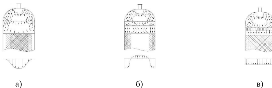
Рисунок 1 – Сравнение распределения скоростей потоков при использовании различных распределительных устройств:
